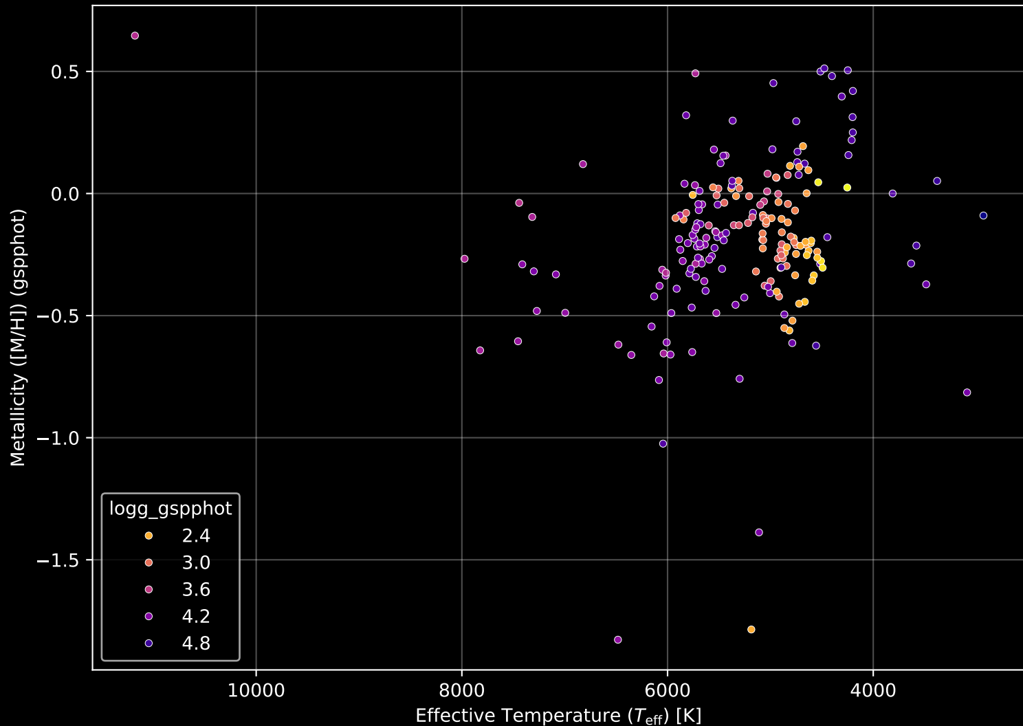
APOGEE DR17 Field: [180+31_MGA] Stellar Population Parameters (n= 208)
